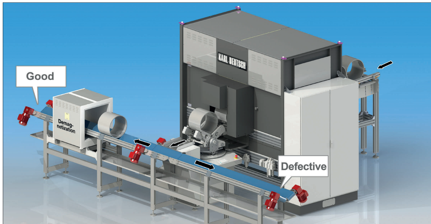
Система контроля муфт с возможностью отбраковки прошедших и не прошедших контроль деталей
